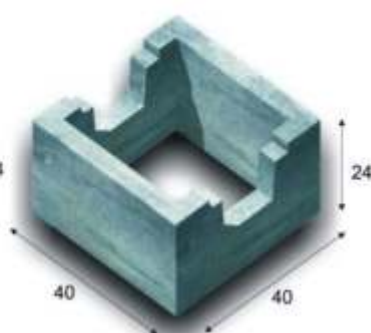
D2 - PUSTAK Z WPUSTEM 40X40X24 cm
