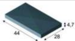
E1 - DASZEK (czterospadowy) 44x28x4,7 cm kolorystyka: grafit, czerwony, brąz waga elementu: 10,30 kg CENA JEDNEGO ELEMENTU:
