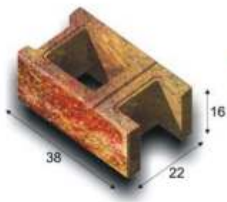
A1 - PUSTAK ŁUPANY (podmurówka) kolorystyka: złota jesień D1 i D2 waga elementu: 19,20 kg ilość w pakiecie: CENA JEDNEGO ELEMENTU: ZŁOTA JESIEŃ D1, D2 -
