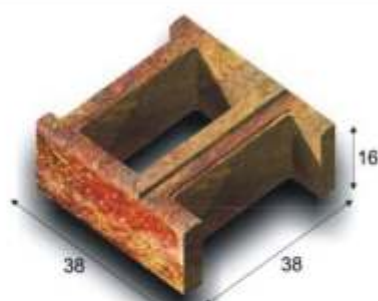
B1 - PUSTAK ŁUPANY (podmurówka) kolorystyka: złota jesień D1 i D2 waga elementu: 25,50 kg ilość w pakiecie: sprzedawany w komplecie CENA JEDNEGO ELEMENTU: ZŁOTA JESIEŃ D1, D2 -
