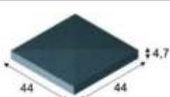
E3 - DASZEK (czterospadowy) 44x44x4,7 cm kolorystyka: grafit, czerwony, brąz waga elementu: 17,00 kg CENA JEDNEGO ELEMENTU:
