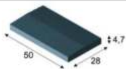
E2 - DASZEK (dwuspadowy) 50x28x4,7 cm kolorystyka: grafit, czerwony, brąz waga elementu: 13,30 kg CENA JEDNEGO ELEMENTU:
