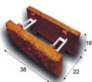
A3 - KSZTAŁTKA (podmurówka) kolorystyka: złota jesień D1 i D2 waga elementu: 12 kg ilość w pakiecie: CENA JEDNEGO ELEMENTU: ZŁOTA JESIEŃ D1, D2 -
