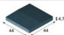
E4 - DASZEK (dwuspadowy) 44x44x4,7 cm kolorystyka: grafit, czerwony, brąz waga elementu: 17,00 kg CENA JEDNEGO ELEMENTU:
